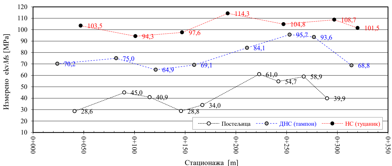
Дијаграм измерених вредности модула стишљивости
