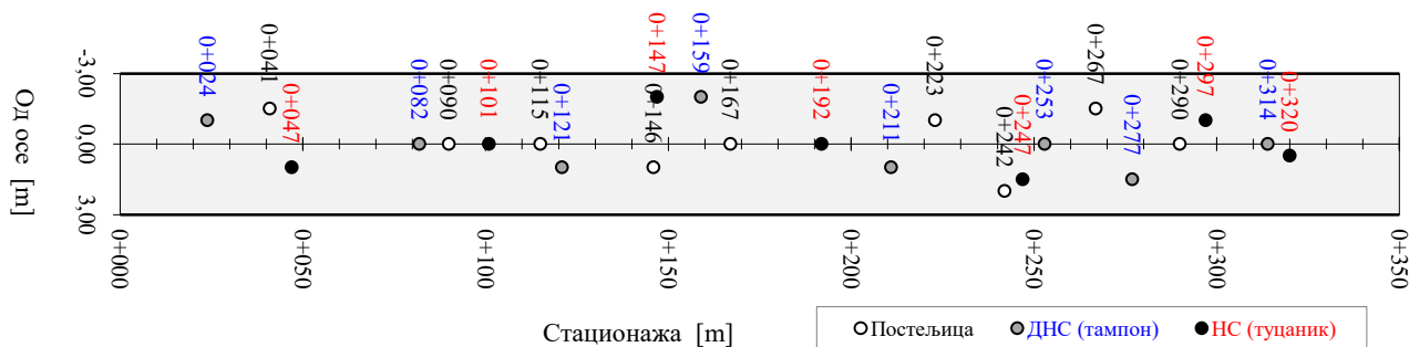
Ситуациона скица са распоредом мерних места
